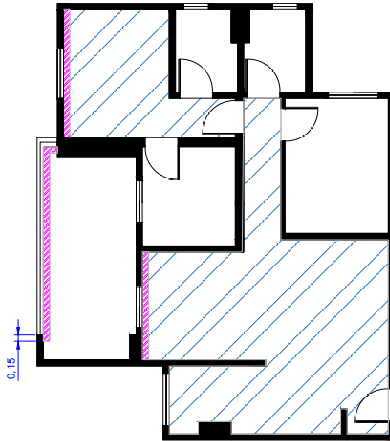
PLANTA DE REBAIXO DE GESSO ESC. 1:75
