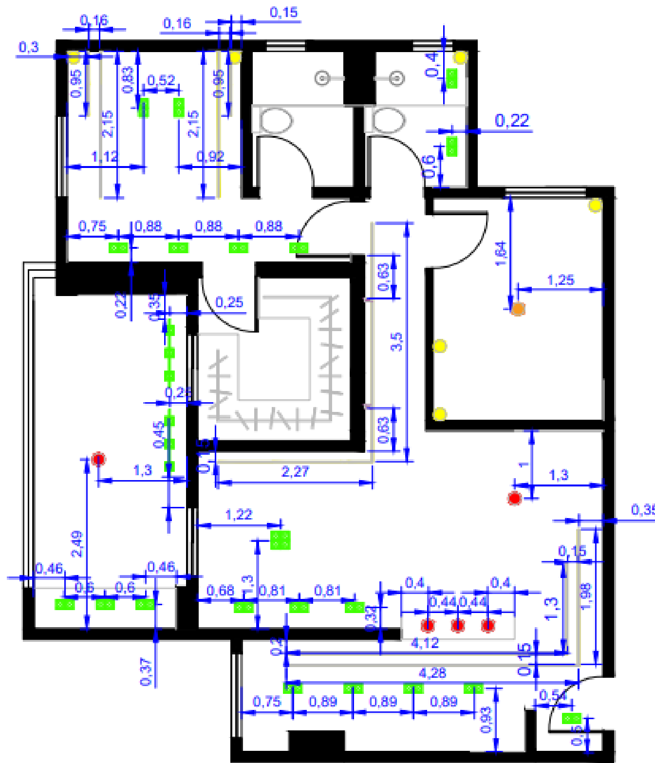
PLANTA DE ELÉTRICA ESC. 1:75
