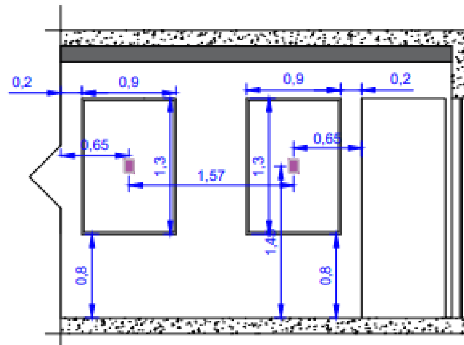
VISTA 01: BOSERIER E ARANDELA ESC. 1:50
