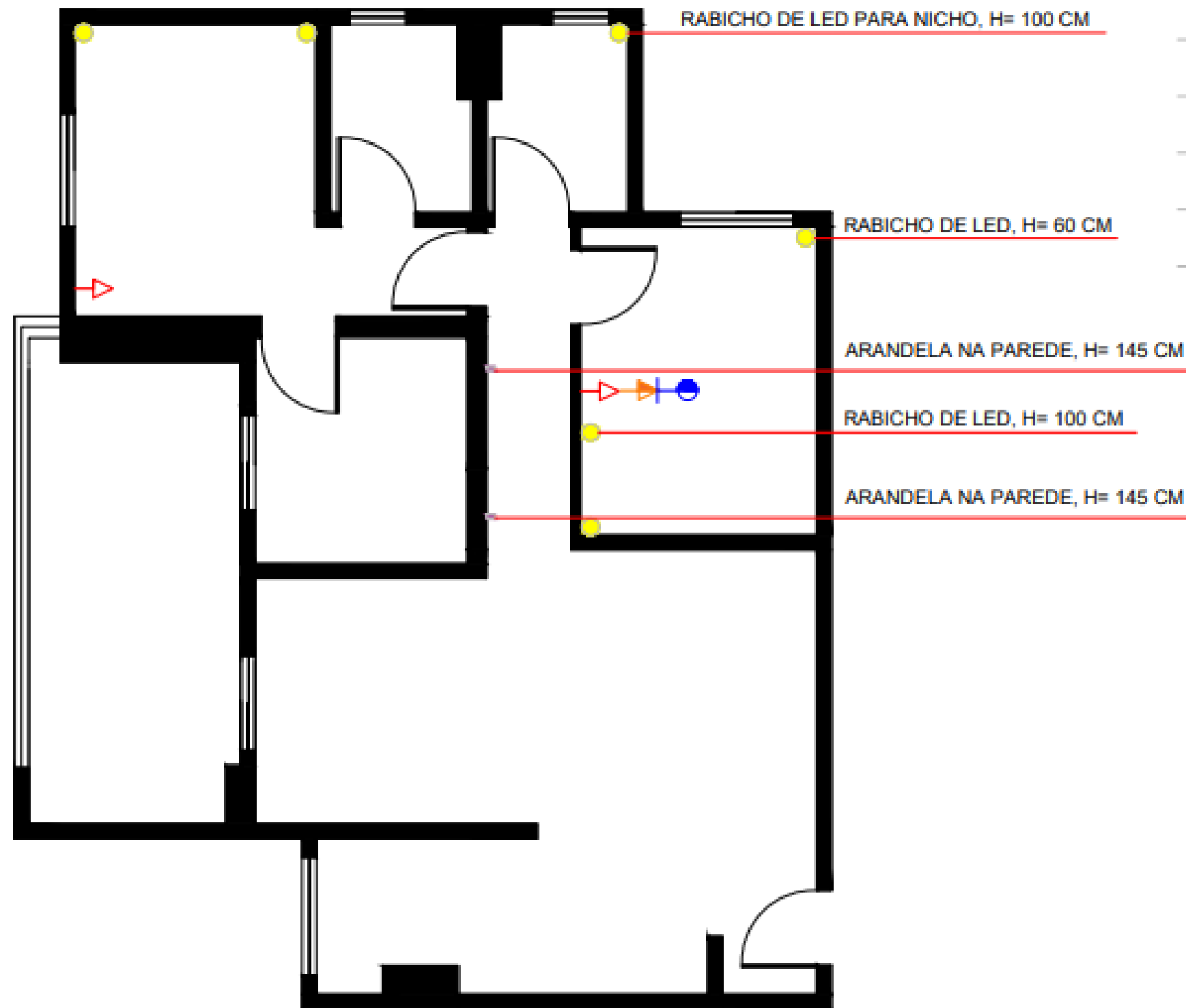
PLANTA DE ELÉTRICA DE PAREDE ESC. 1:75
