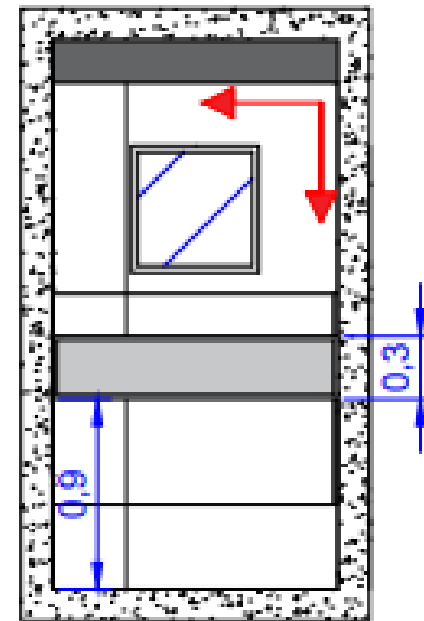
VISTA 02: W.C SOCIAL ESC. 1:50
