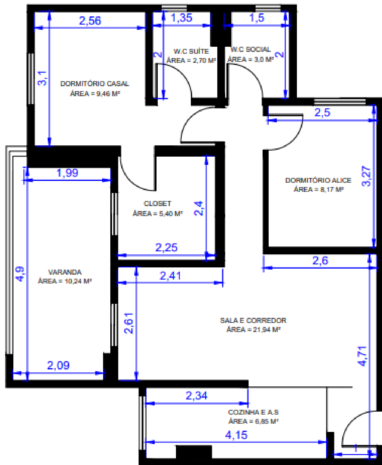
PLANTA DE MEDIDAS GERAIS ESC. 1:75
