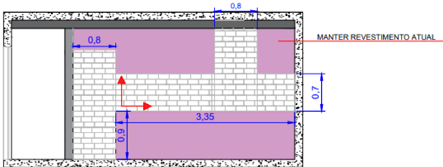
VISTA 03: COZINHA E A.S ESC. 1:50
