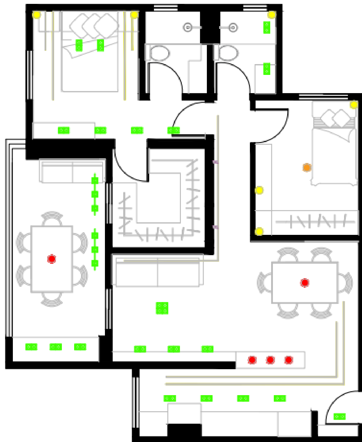
PLANTA DE LAYOUT E ELÉTRICA ESC. 1:75
