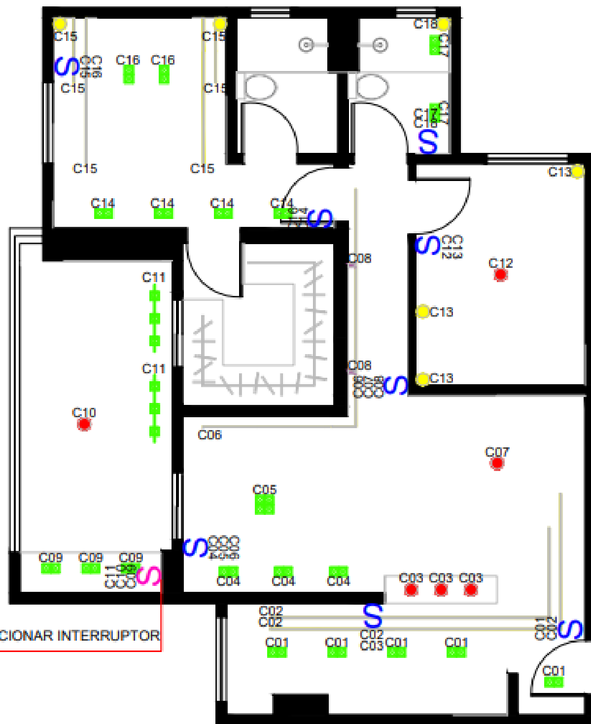
PLANTA DE CIRCUITO ESC. 1:75
