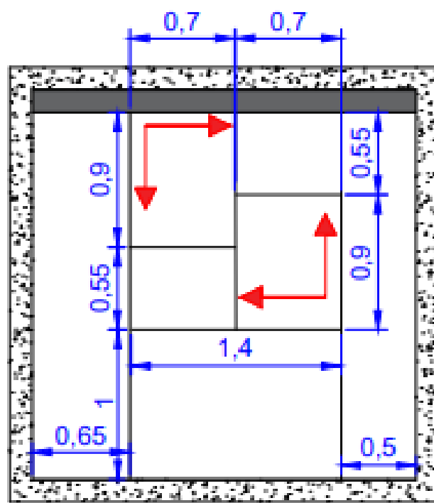
VISTA 01: CABECEIRA CAMA ESC. 1:50
