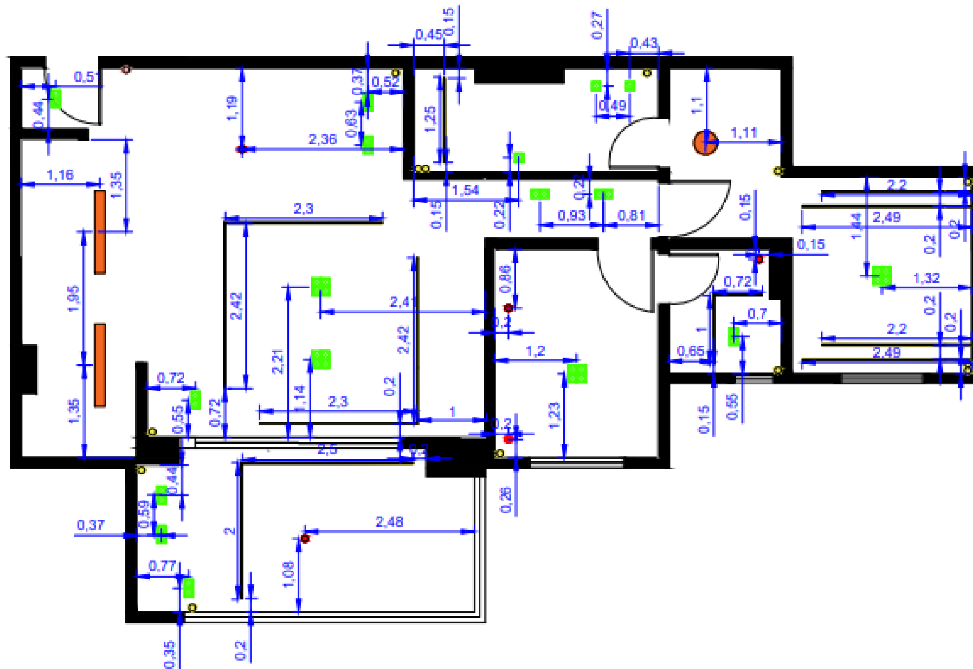
PLANTA DE ELÉTRICA DE TETO ESC. 1:75
