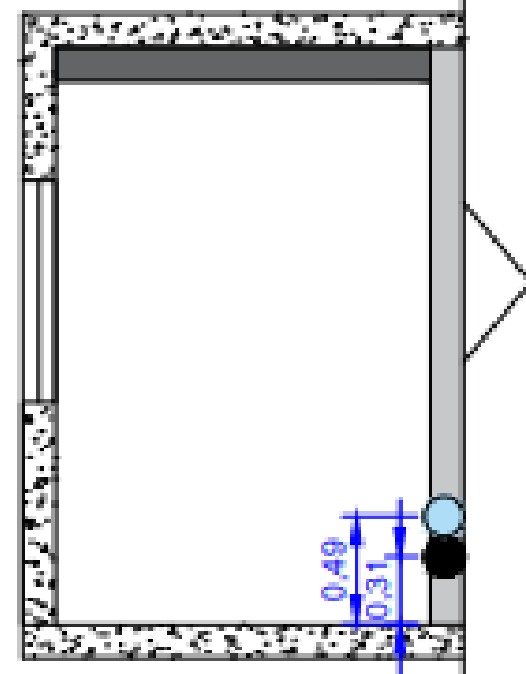
VISTA 02 - PONTOS DE HIDRÁULICA PARA MÁQUINA LAVA LOUÇA ESC: 1:50
