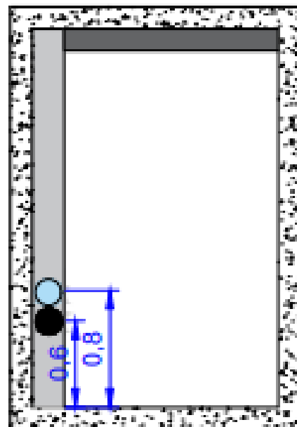
VISTA 01 - PONTOS DE HIDRÁULICA A.S. ESC: 1:50
