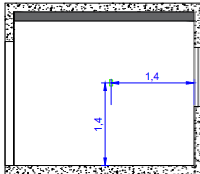
VISTA 02 - SUÍTE 02 ESC. 1:50
