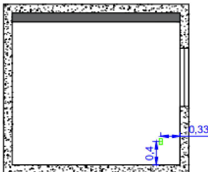
VISTA 04 - SUÍTE PRINCIPAL ESC. 1:50
