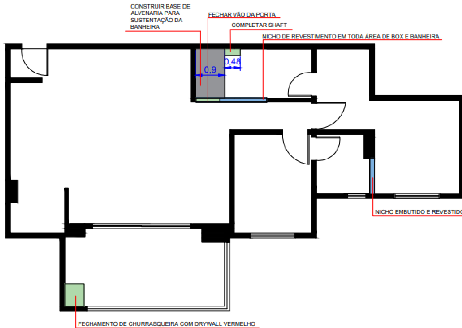
PLANTA DE CONSTRUIR ESC. 1:75
