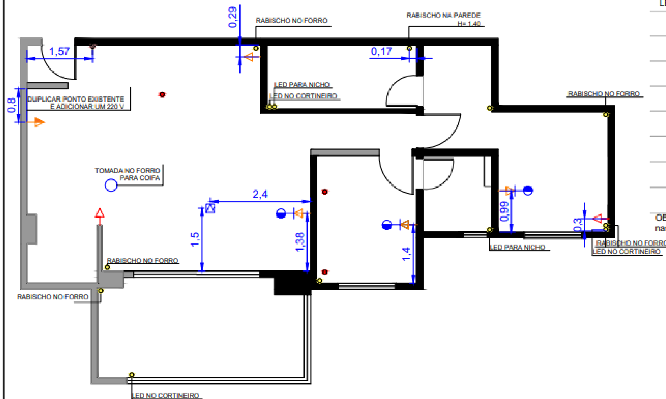
PLANTA DE ELÉTRICA DE PAREDE ESC. 1:75
