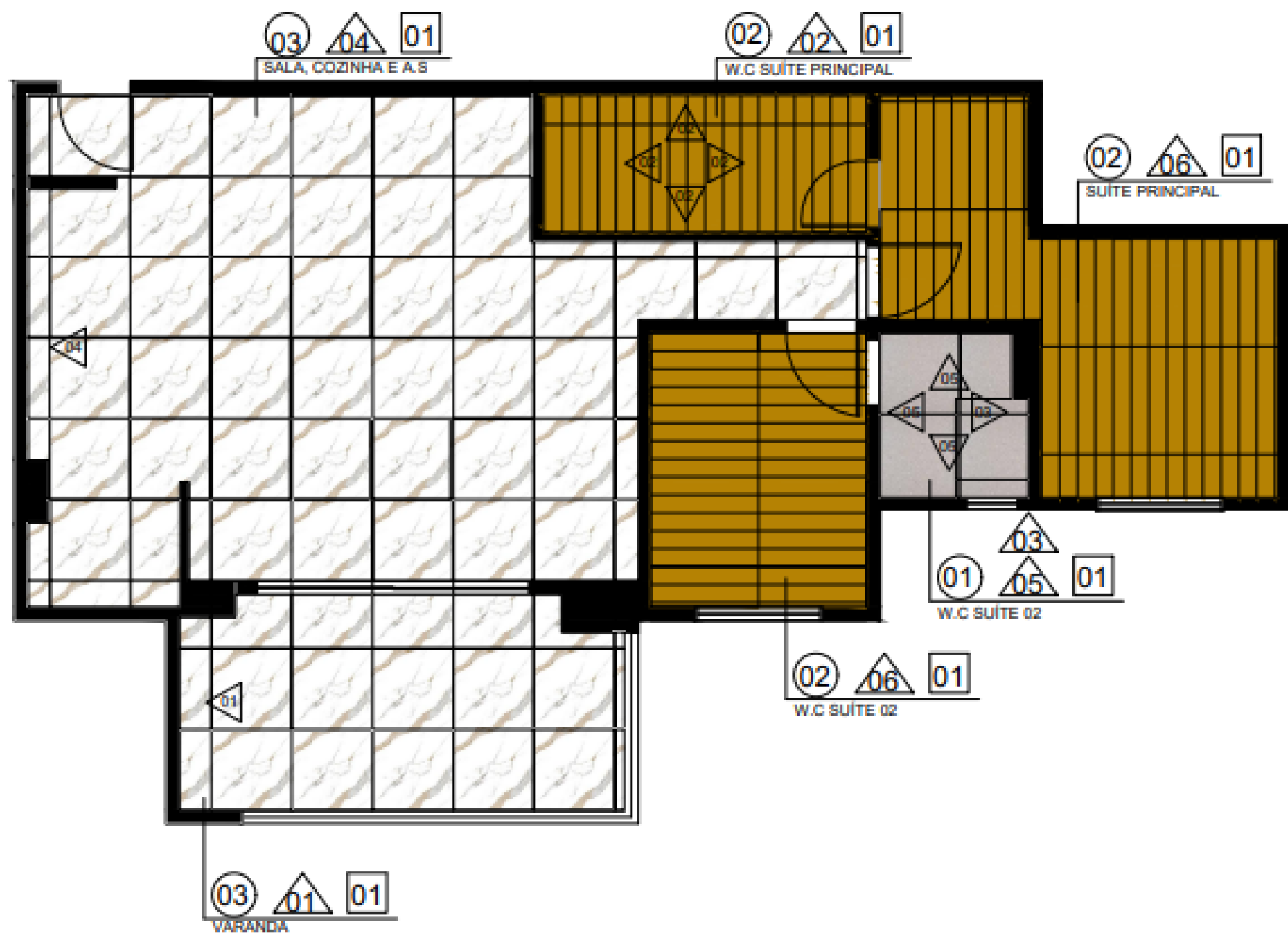
PLANTA DE PAGINAÇÃO DE PISO ESC. 1:75
